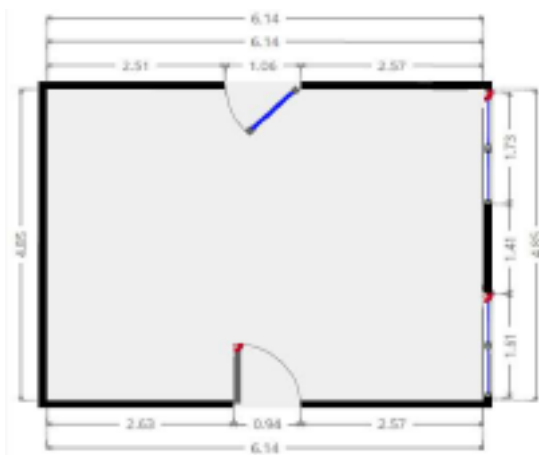
Beispiel Grundriss
